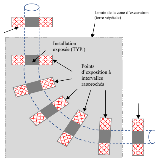
Schéma 16: Points d'exposition pour les coudes
