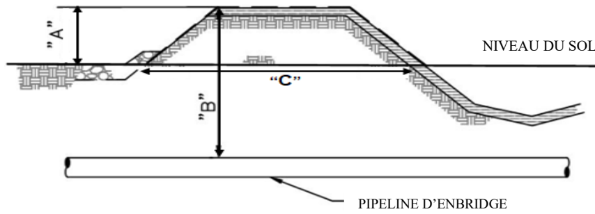
Schéma 11: Bermes mineures – dessin type
