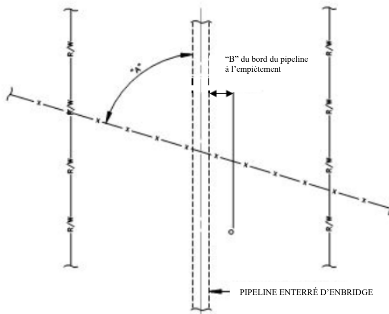
Schéma 12: Installations en surface – dessin type
