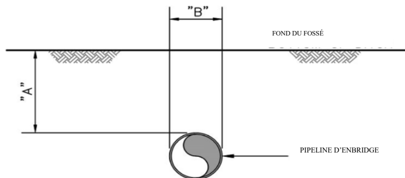
Schéma 10: Restauration du fossé — dessin type
