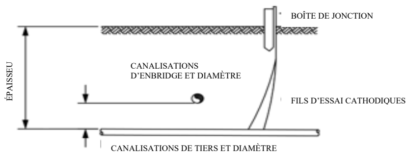
Schéma 4: Connexion du fil d'essai pour un pipeline en acier – dessin type
