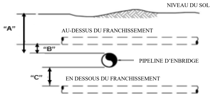
Schéma 3: Franchissement d'installation – dessin type
