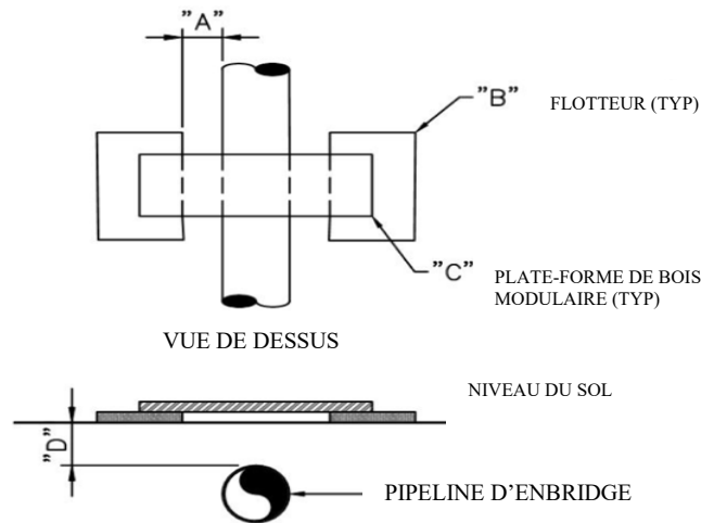
Schéma 8: Ponts passant au-dessus d'un pipeline — dessin type
