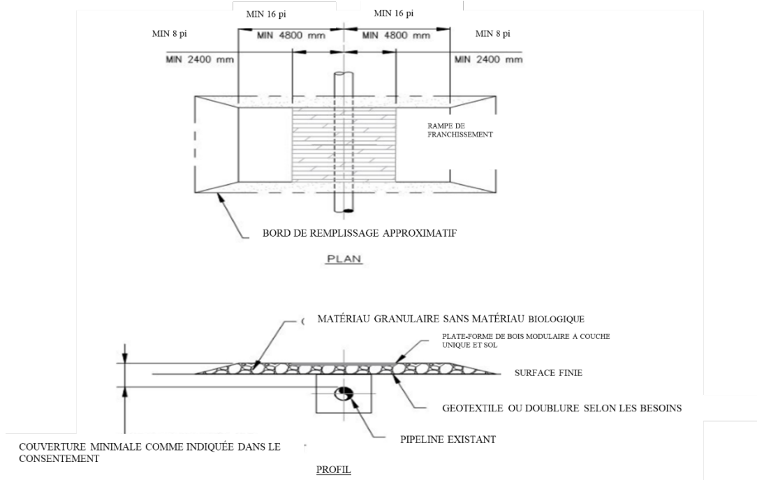
Schéma 7: Rampe de franchissement avec plate-forme de bois modulaire – dessin type
