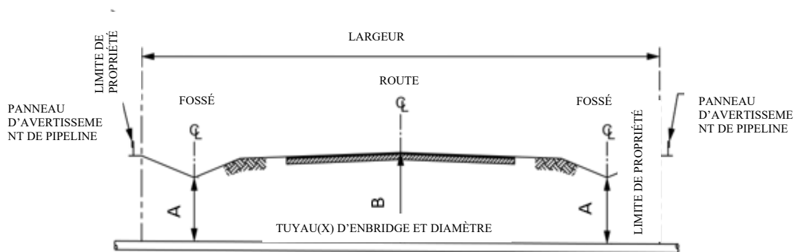
Schéma 2: Franchissement de route — dessin type
