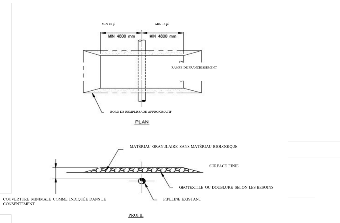
Schéma 6: Rampe de franchissement – dessin type
