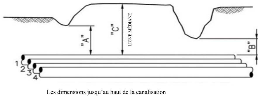
Schéma 9: Resurfacement ou renouvellement du gravelage — dessin type
